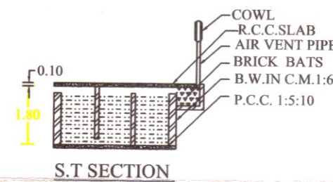
S.T SECTION
