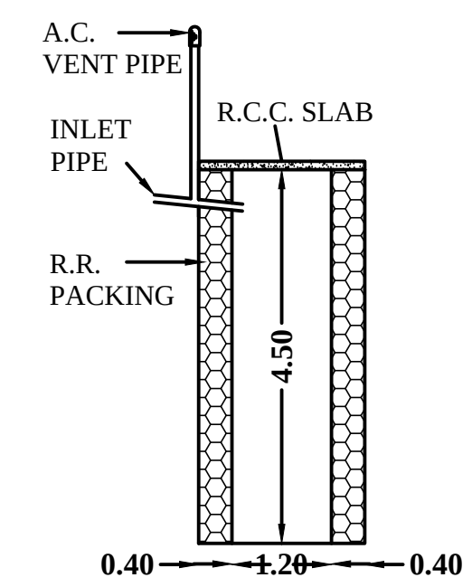
SOAK PIT
