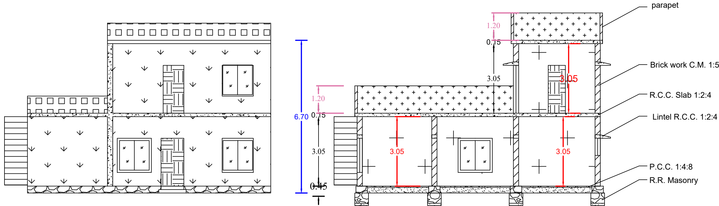
ELEVATION
