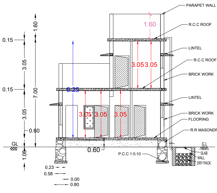
ELEVATION
