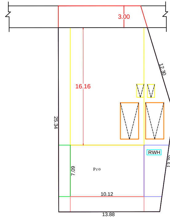
SCALE 1:100 SITE PLAN
