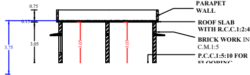
ELEVATION
