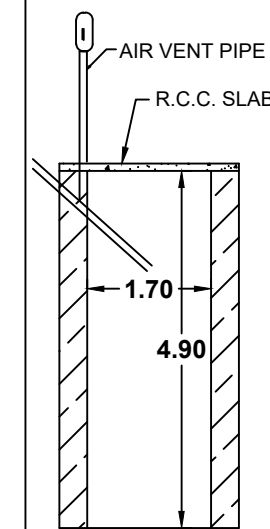
SOAK PIT
