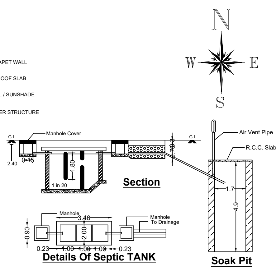
Soak Pit
