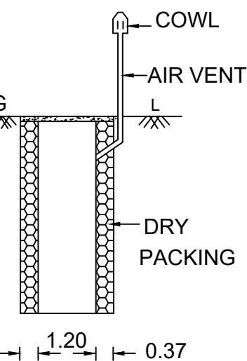
SOAK PIT
