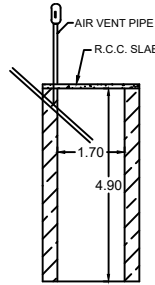
SOAK PIT
