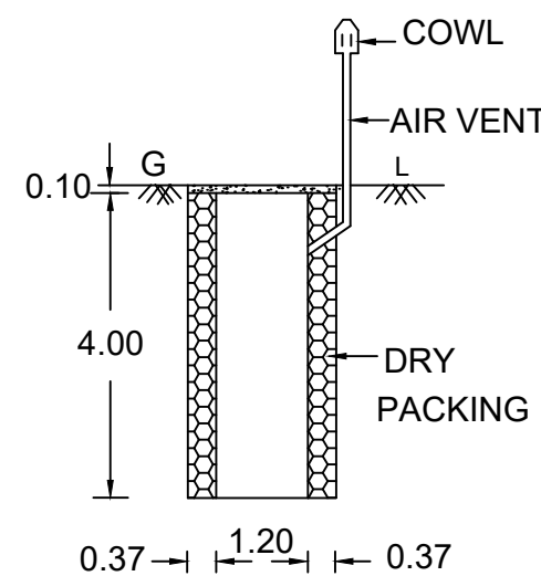
SOAK PIT
