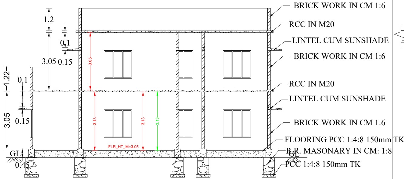
SECTION A-A
