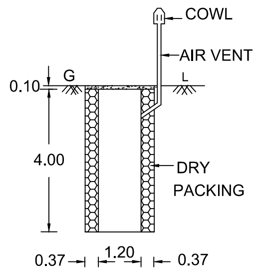
SOAK PIT
