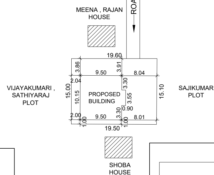
KEY PLAN Scale : 1:400
