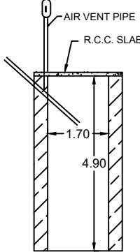
SOAK PIT
