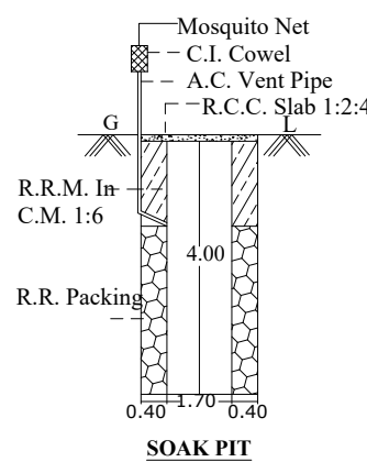
SOAK PIT
