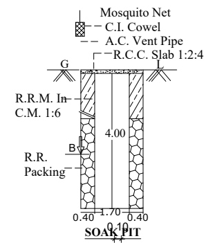
SOAK PIT
