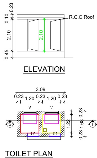
TOILET PLAN
