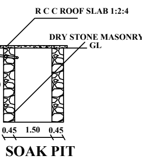
SOAK PIT
