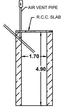
SOAK PIT
