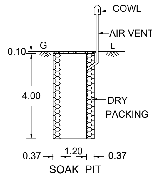
SOAK PIT
