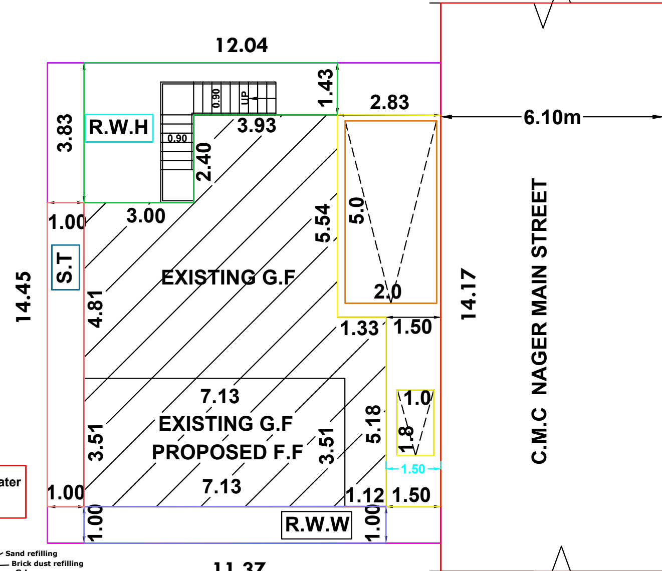
11.37 SITE PLAN SCALE 1:100
