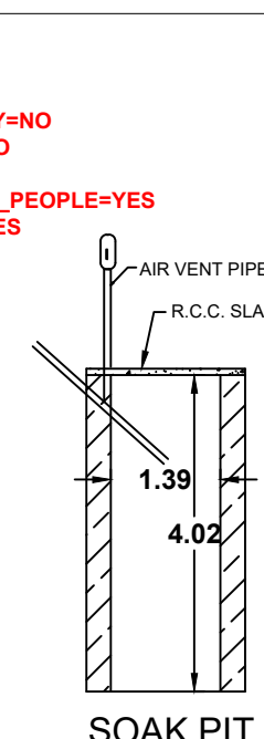
SOAK PIT
