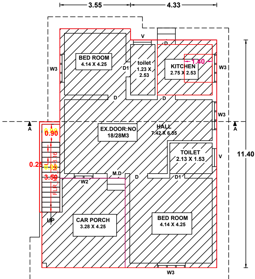
G. FLOOR PLAN
