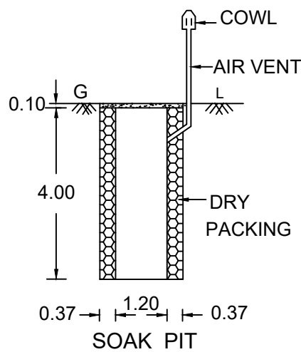
SOAK PIT
