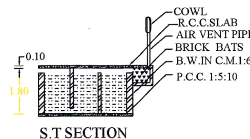
S.T. SECTION
