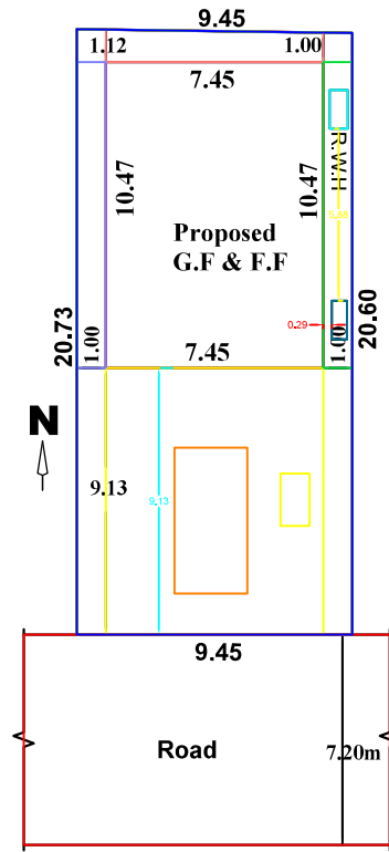
SITE PLAN SCALE 1:100
