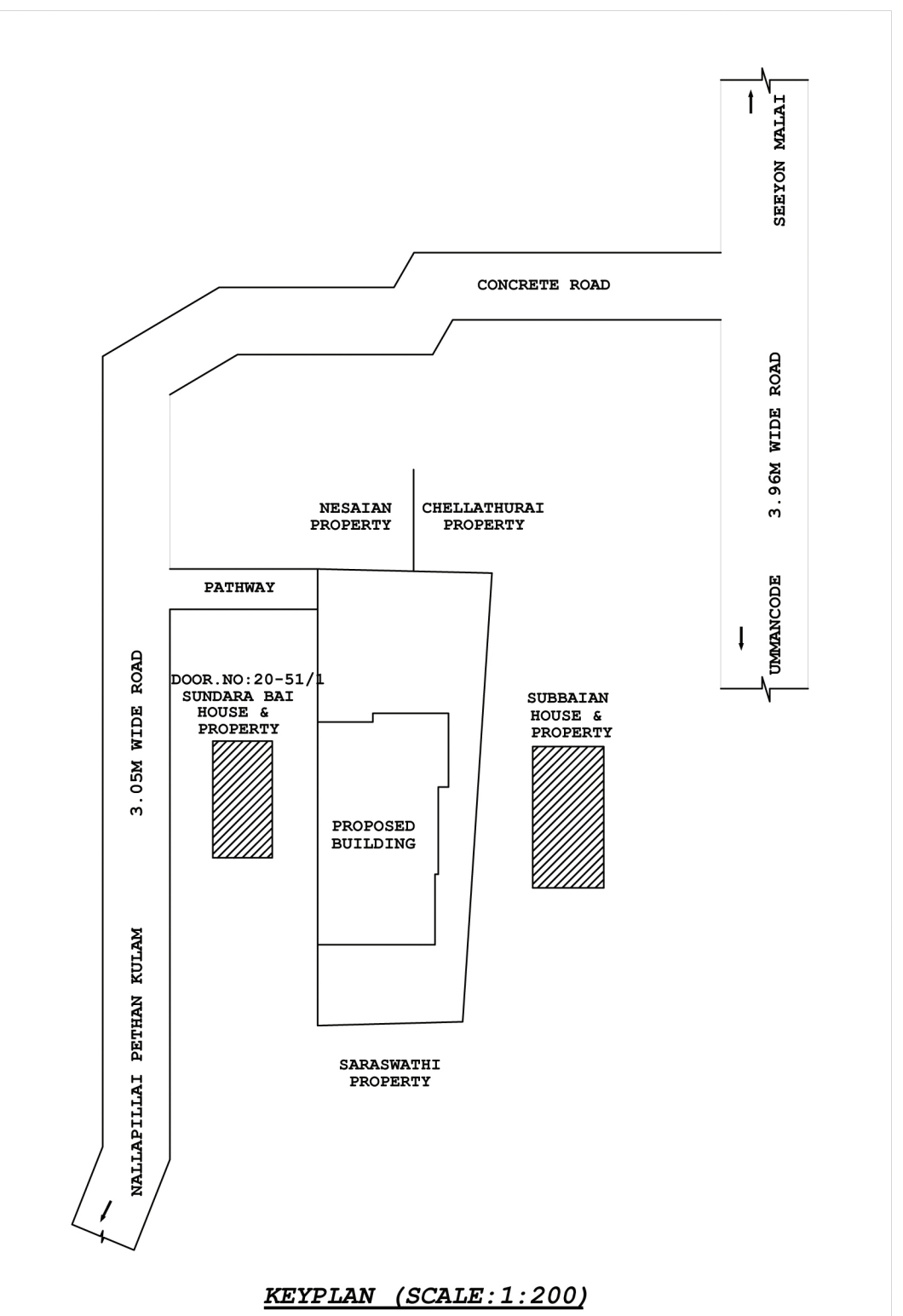
KEYPLAN (SCALE:1:200)
