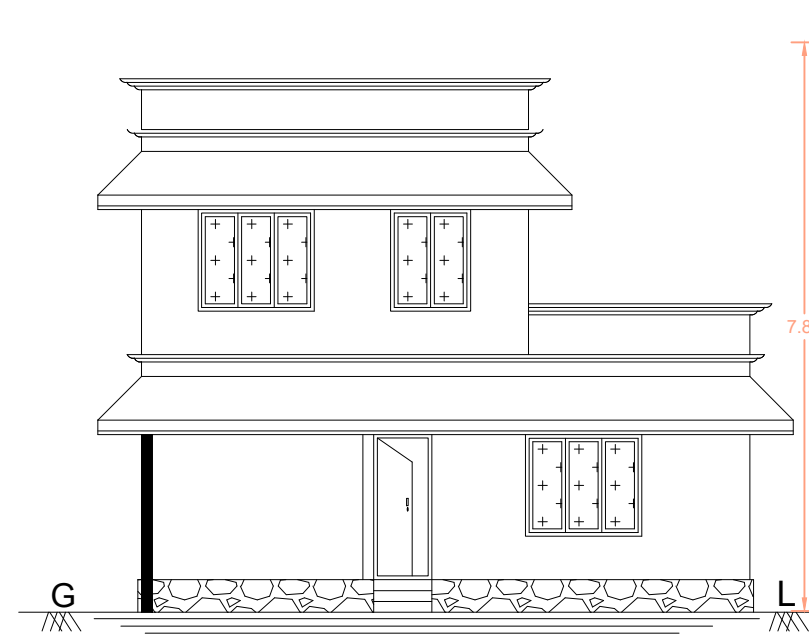
ELEVATION
