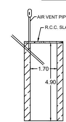
SOAK PIT
