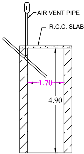
SOAK PIT
