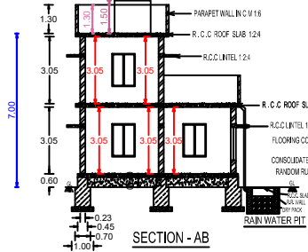
SECTION - AB
