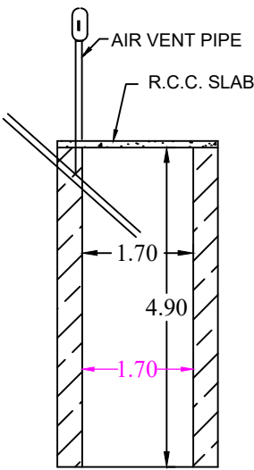
SOAK PIT
