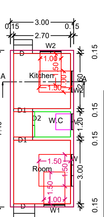
G. FLOORPLAN
