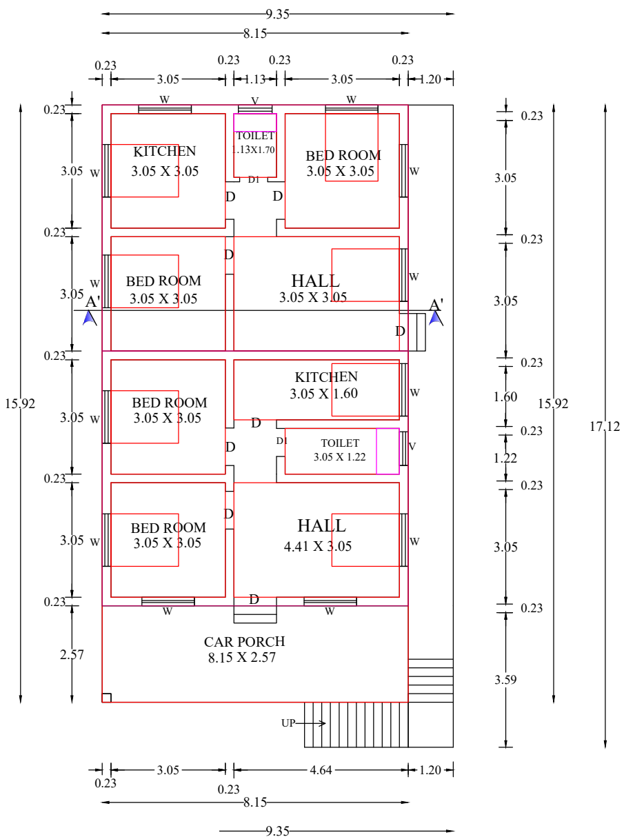
UND FLOOR
