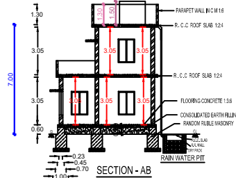
SECTION - AB
