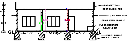
SECTION -AB
