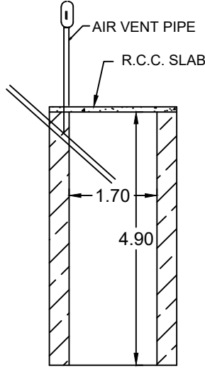
SOAK PIT
