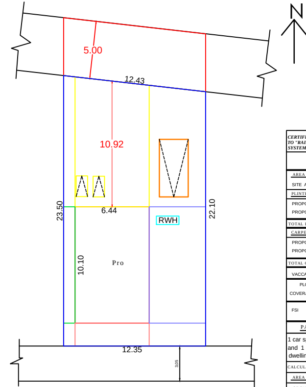
SCALE 1:100 SITE PLAN
