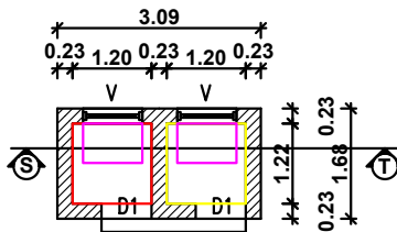
TOILET PLAN
