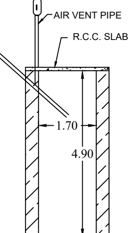
SOAK PIT
