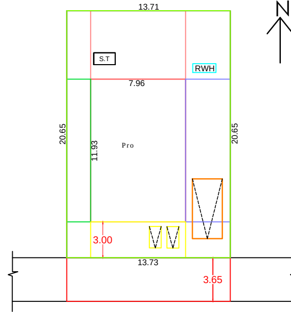
SCALE 1:100 SITE PLAN
