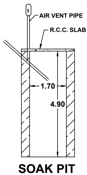
SOAK PIT
