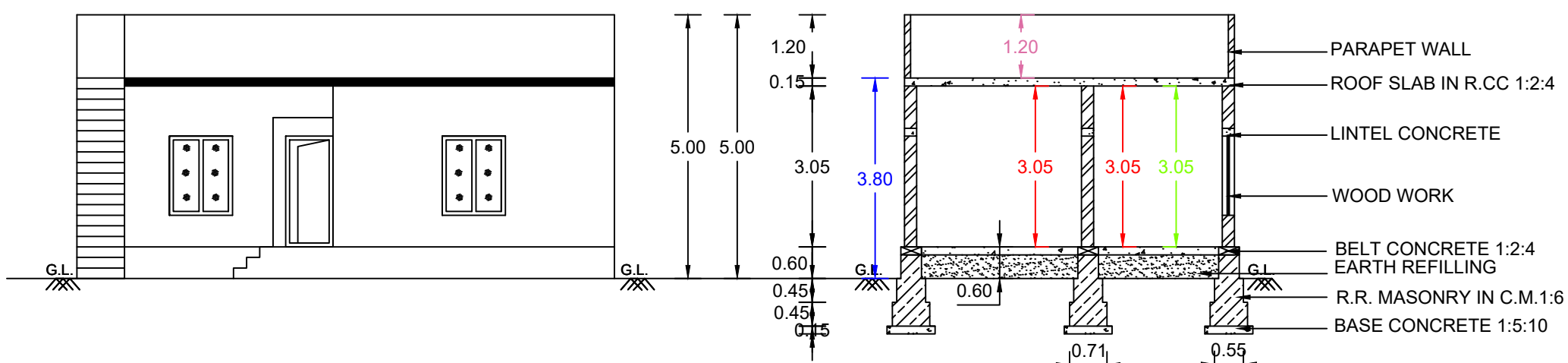
ELEVATION
