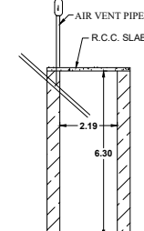
SOAK PIT
