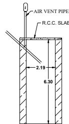
SOAK PIT
