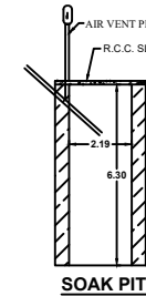
SOAK PIT
