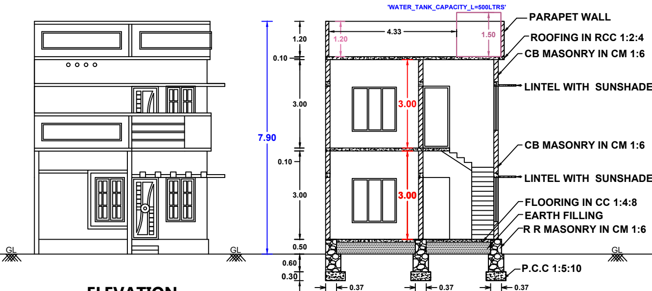
ELEVATION
