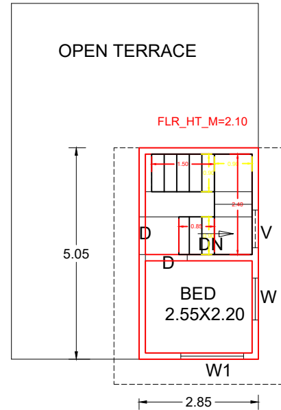
F.F. PLAN
