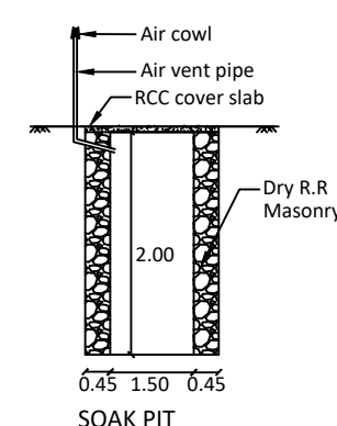
SOAK PIT
