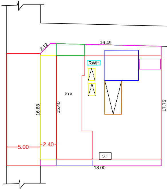
SCALE 1:100 SITE PLAN
